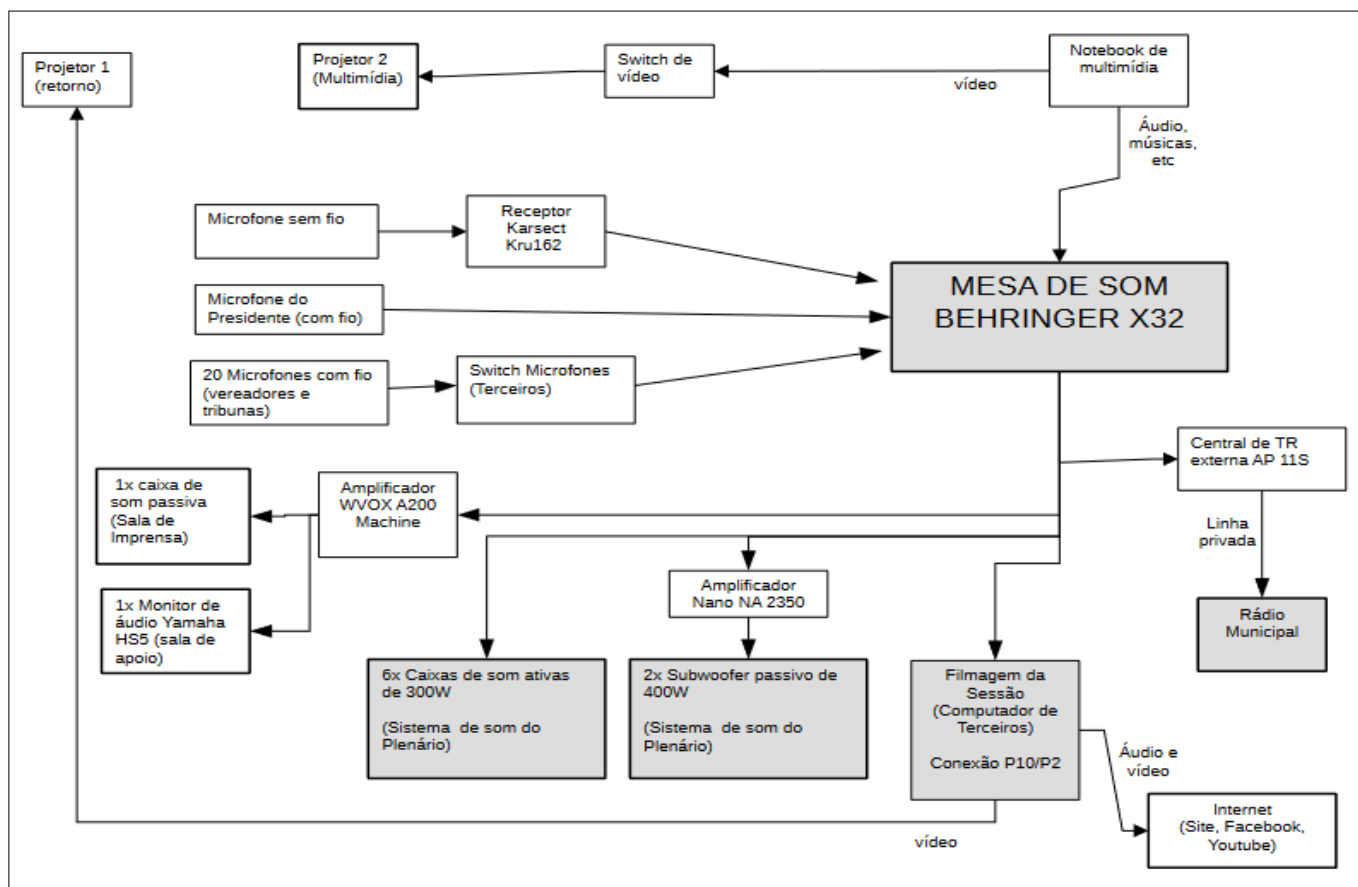
Figura 1 – Representação do sistema de áudio – Plenário Dr. Tancredo Neves
