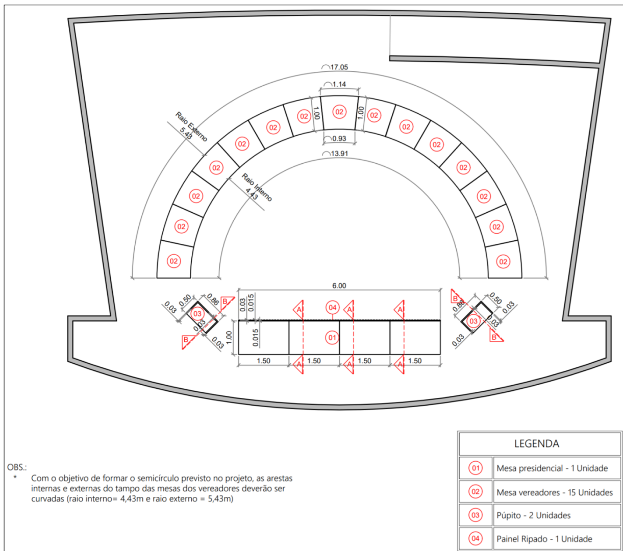
Imagem 1.3. - Vista superior – Dimensões de topo e Cortes
