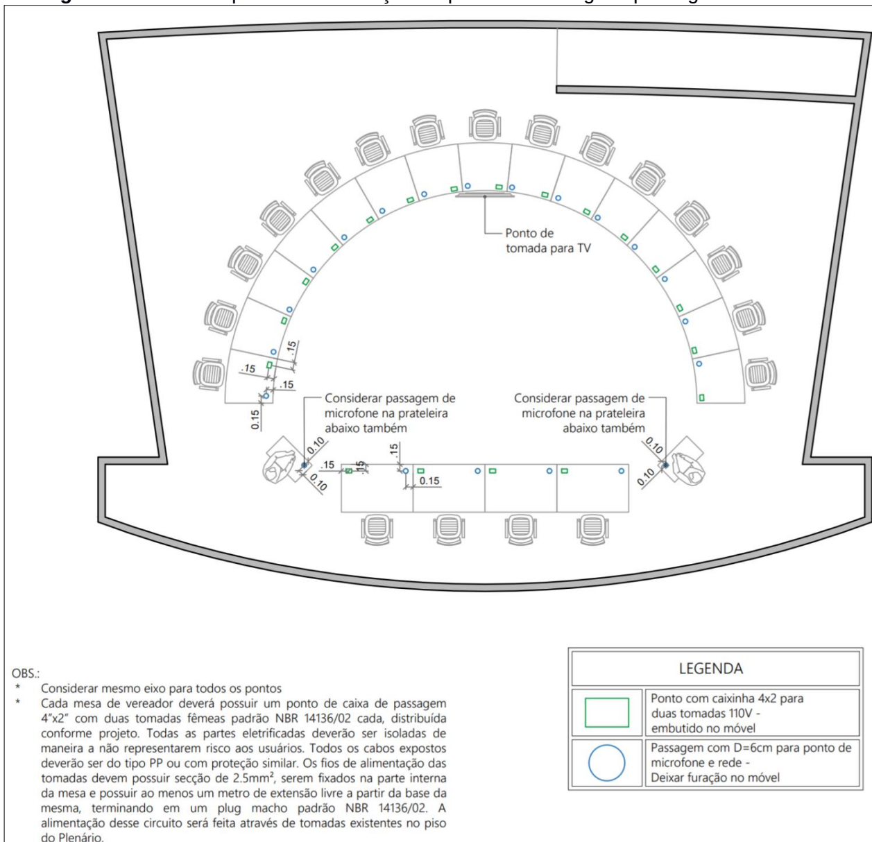
Imagem 1.2. - Vista superior – Localização de pontos de energia e passagem de cabos
