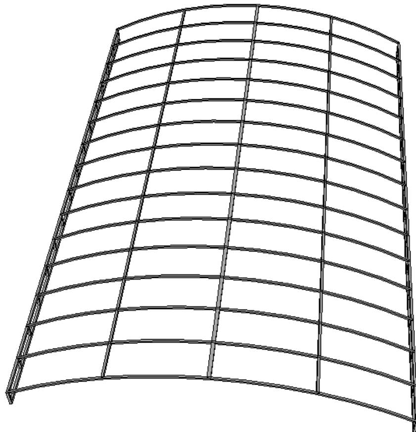
Imagem 11. Estrutura da lona e vigas de apoio – sem tesouras e pilares – vista superior.
