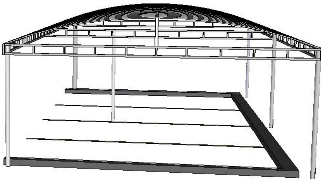
Imagem 14. Referência – Estrutura metálica da cobertura das vagas 1 até 4 – vista lateral direita.
