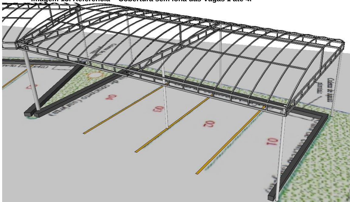
Imagem 14. Referência – Estrutura metálica da cobertura das vagas 1 até 4 – vista lateral direita.
