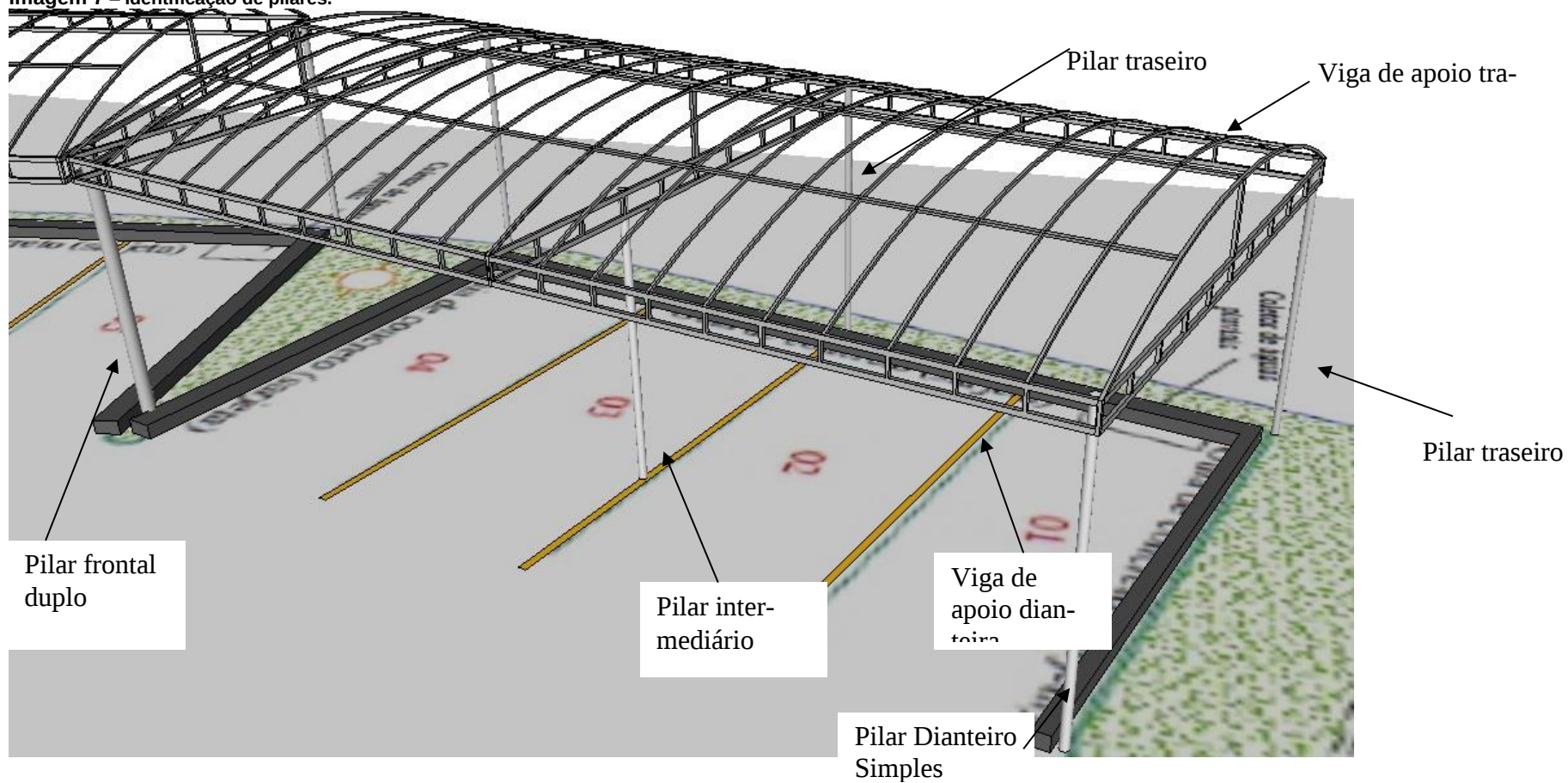
Imagem 7 – Identificação de pilares.
