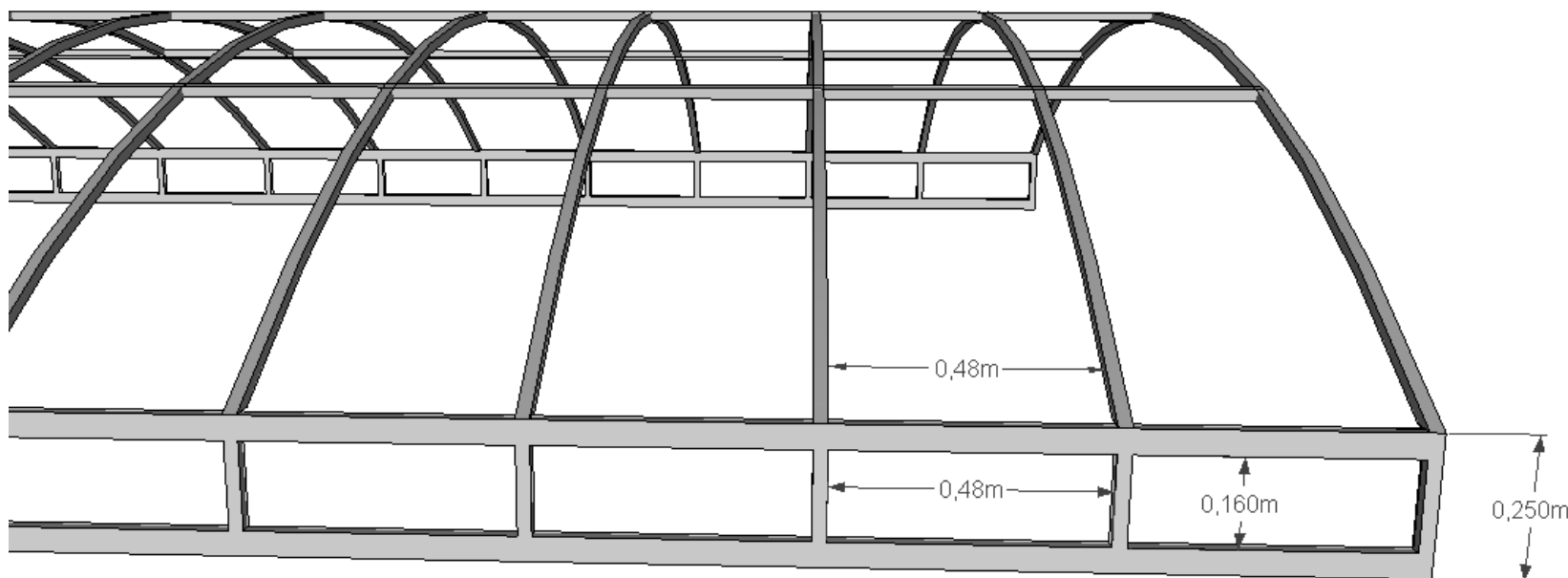
Imagem 12. Estrutura da lona e vigas de apoio – sem tesouras e pilares – dimensões.
