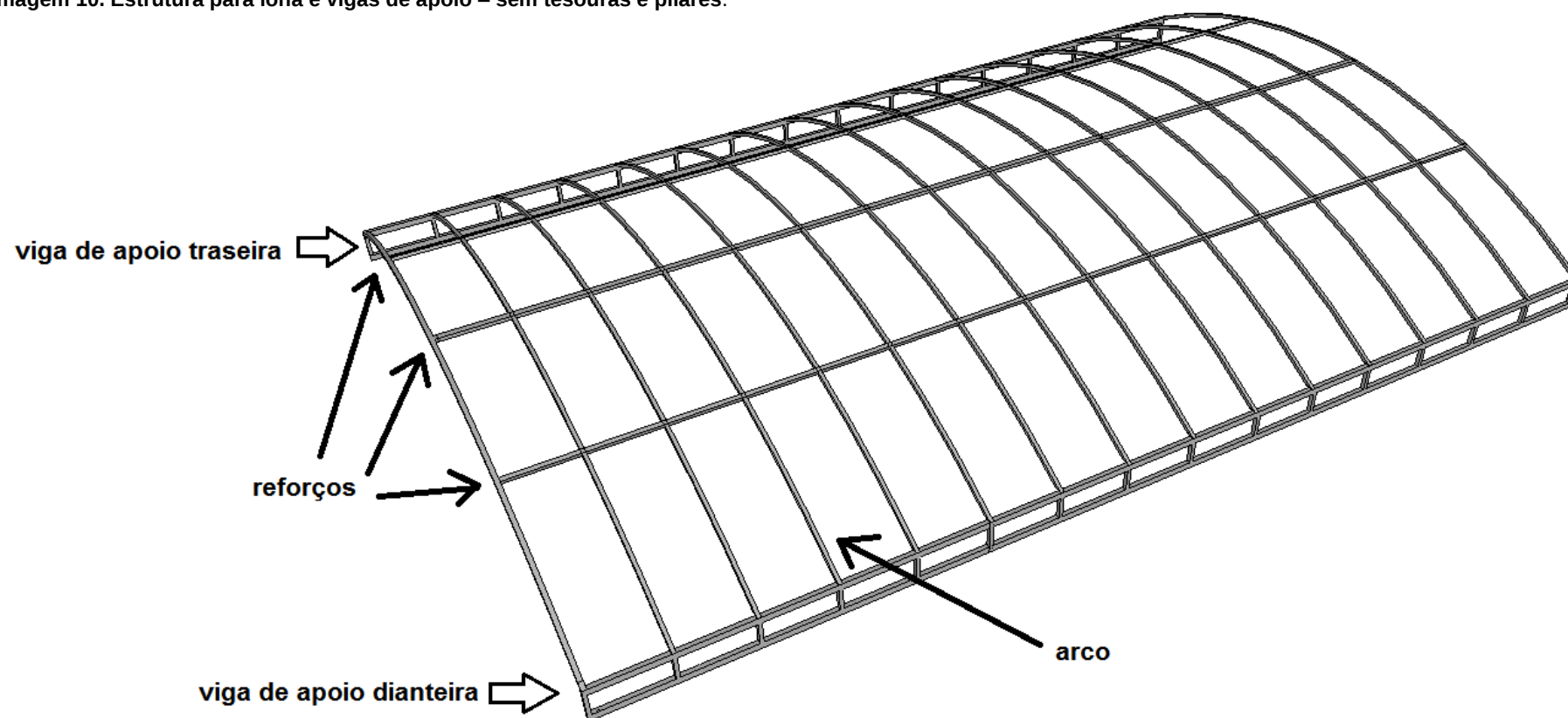
Imagem 10. Estrutura para lona e vigas de apoio – sem tesouras e pilares.
