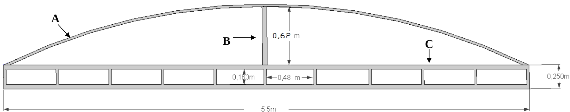
Imagem 6 – Representação lateral das tesouras/vigas.
